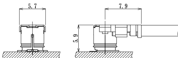
勘合図
