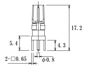
Receptacle DM537R-PC
