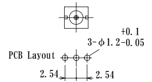
Receptacle DM537R-PC-L2
