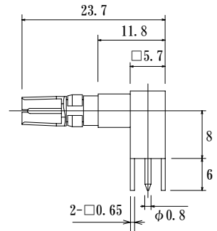
Receptacle DM537R-PC-L2
