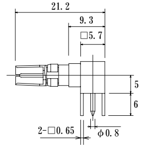
Receptacle DM537R-PC-L1
