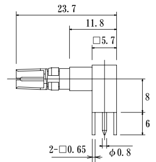
Receptacle DM537R75-PC-L2
